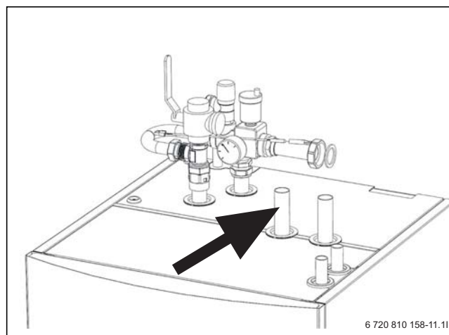
Fig. 18 Påfyldning af radiator og varmesystem skal ske på returledningen til varmepumpen.
