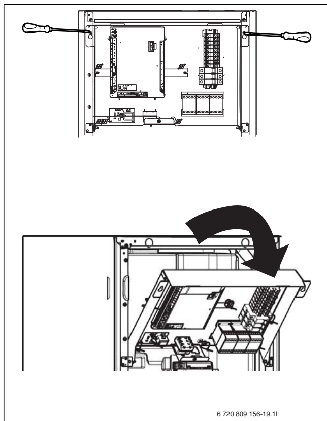
Fig. 36 Sikringsskab
