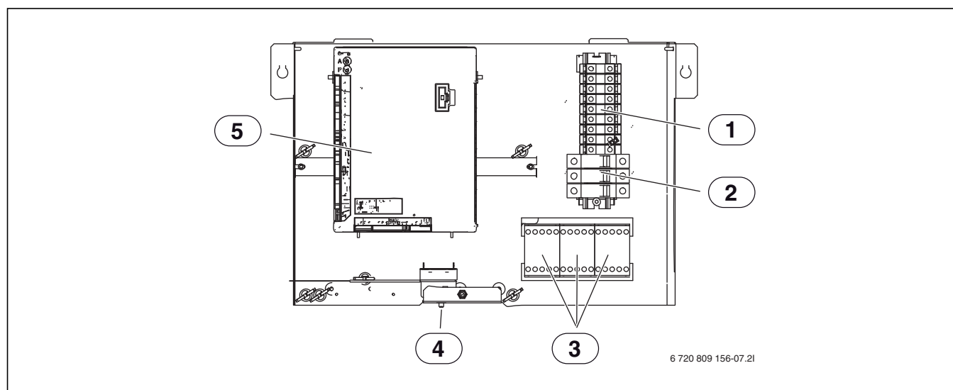
Fig. 23 Layout i styreskab
