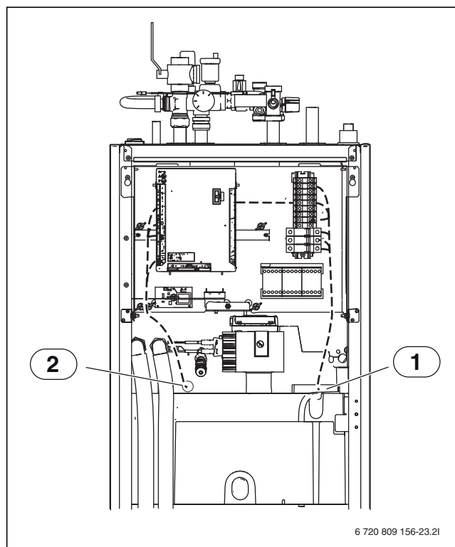
Fig. 22 Kabelgennemføringer
