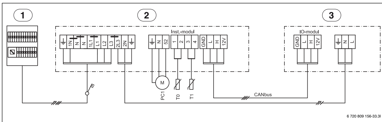
Fig. 27 Tilslutningsdiagram 9kW 3N~
