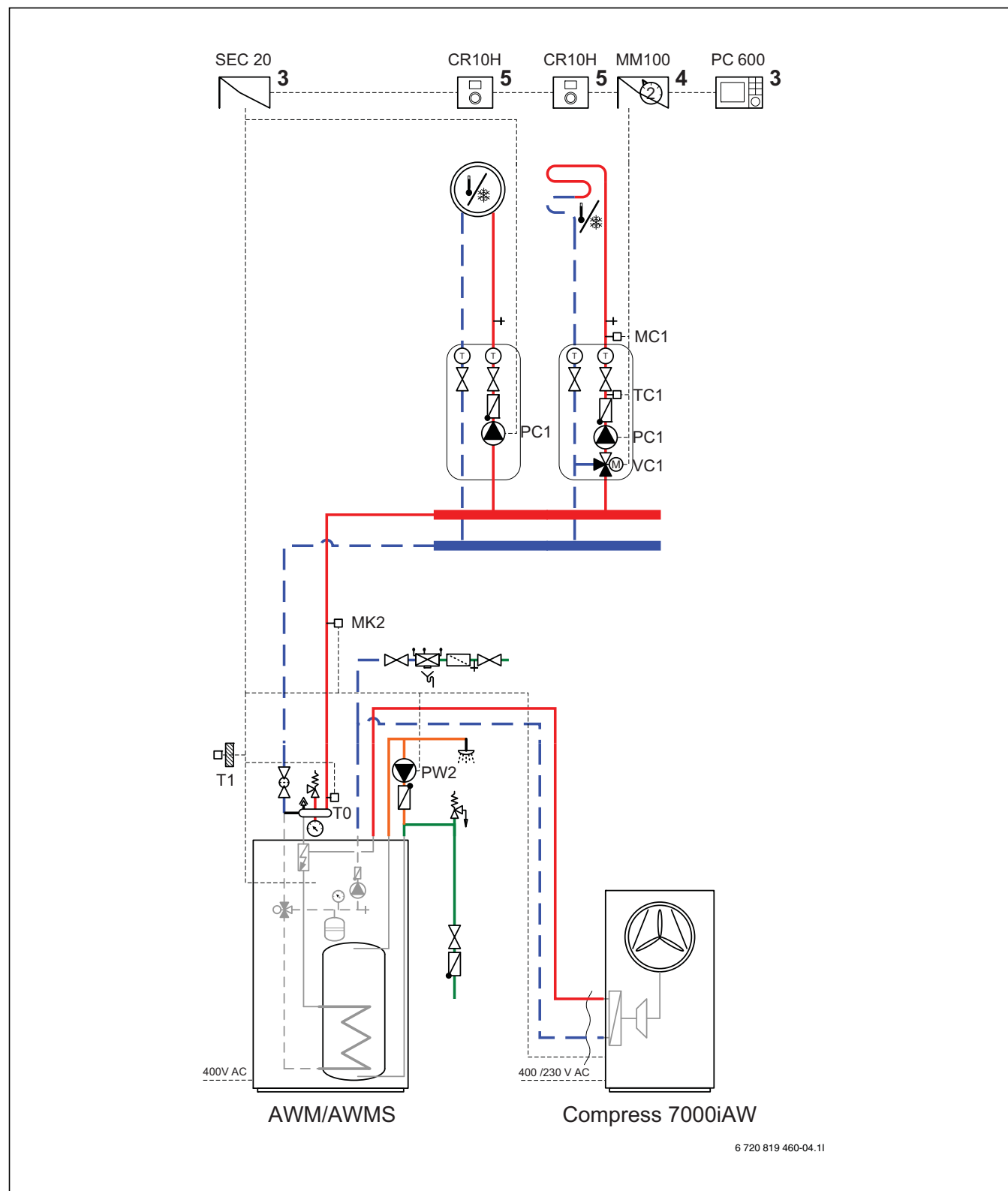
Fig. 4 Varmepumpe med varmepumpemodul
