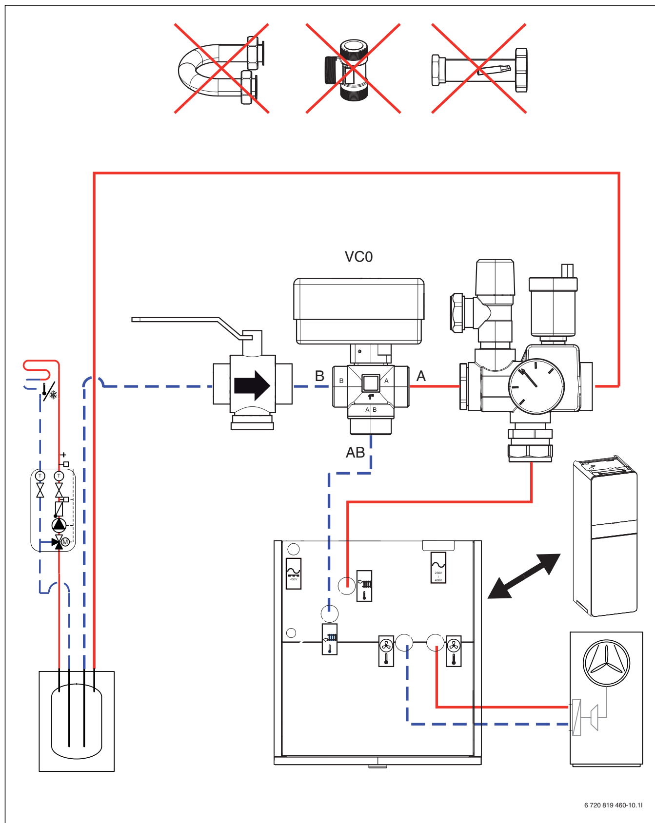
Fig. 43 Installation med buffer tank
