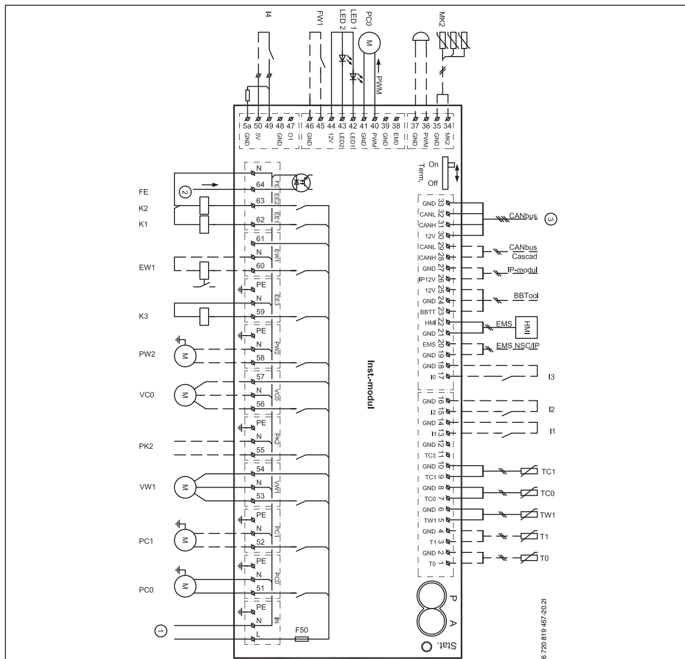
Fig. 32 Strømdiagram, Installationsmodul
