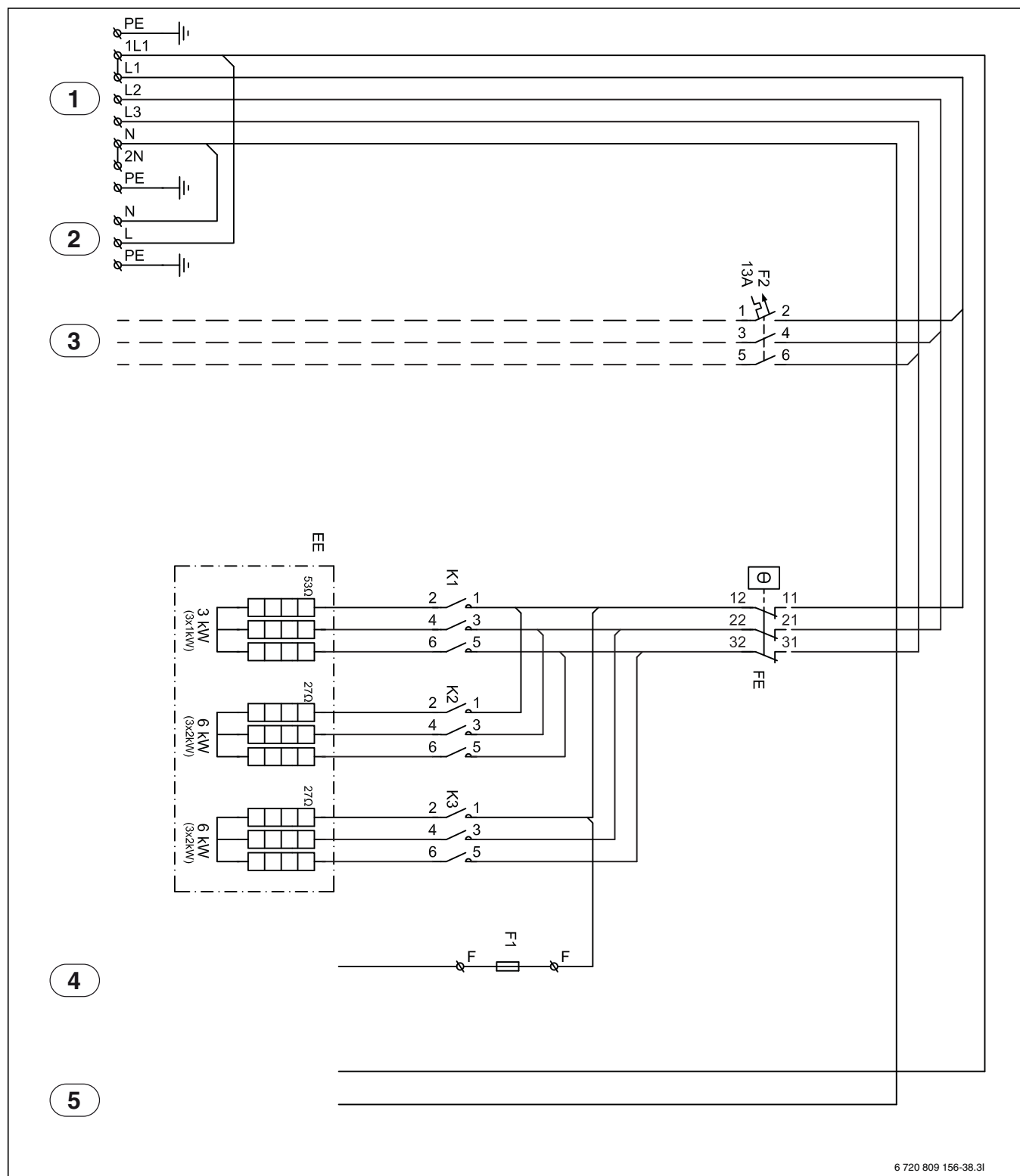
Fig. 31 Elforsyning varmepumpe og varmepumpemodul 15kW
