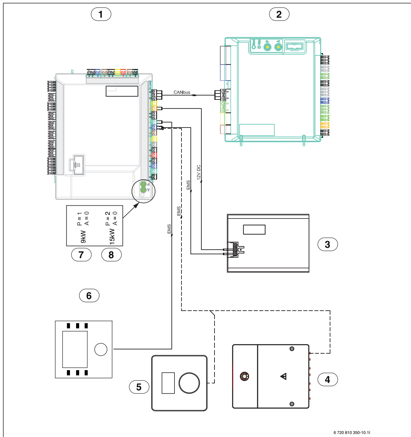
Fig. 33 Kredsdiagram varmepumpe/varmepumpemodul
