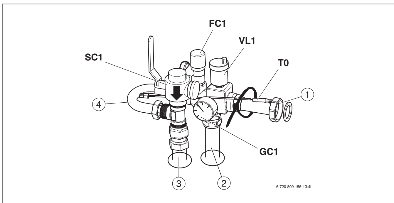
Fig. 11 Sikkerhedsgruppe monteret
