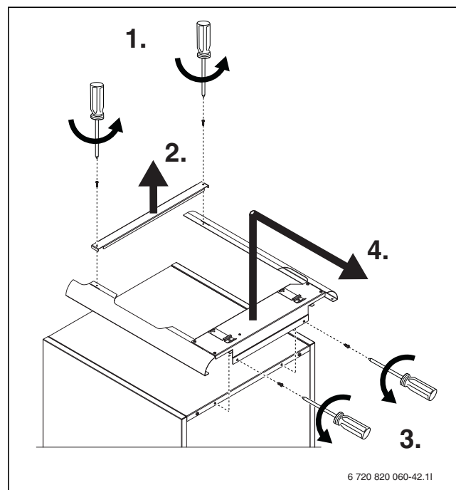
Fig. 13 Fjern tagdele
