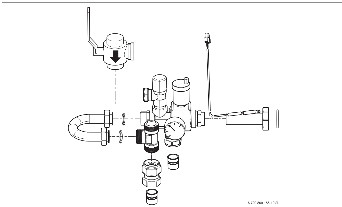
Fig. 10 Sikkerhedsgruppe, leveranceudførelse
