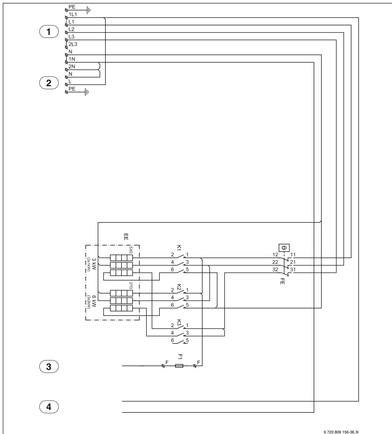
Fig. 30 Elforsyning varmepumpe og varmepumpemodul 9kW
